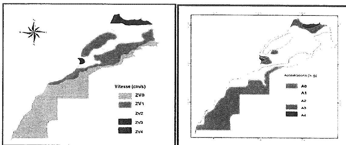
Carte sismique de l'accélération et de la vitesse selon RPS 2011, source direction technique de l'habitat, de l'urbanisme et de l'aménagement de l'espace
